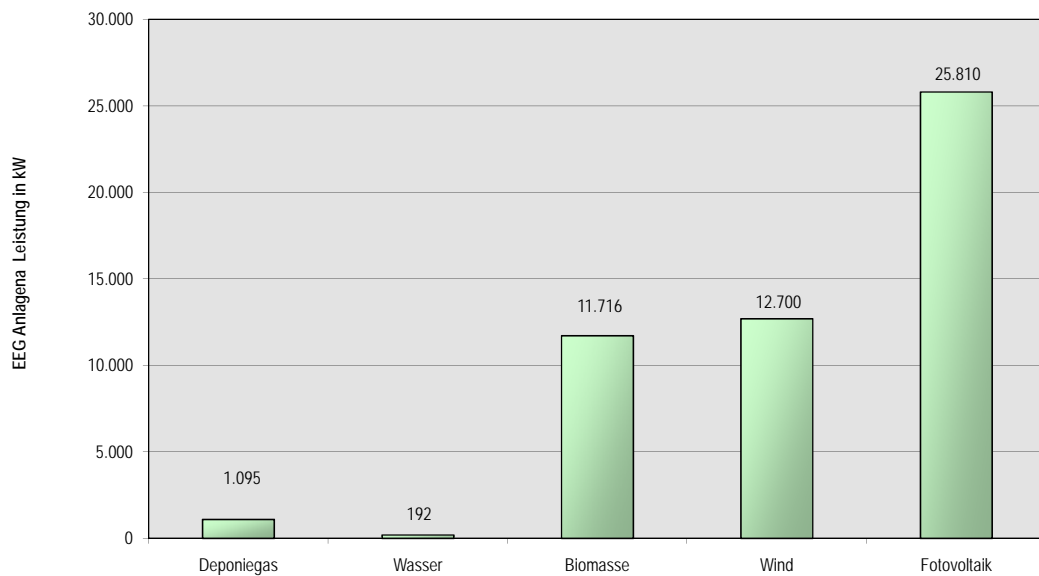
EEG-Anlagen im Gebiet der SWE Netz GmbH im Jahr 2011 - Installierte Leistung
